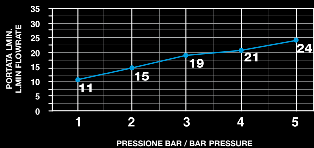
LATO USCITA DOCCIA (*) - Scarico libero a 38° SHOWER OUTLET(*) - 38° waste
